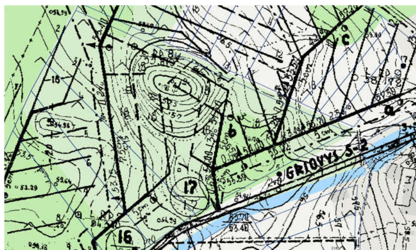
13 pav. Ištrauka iš Melioracijos projekto
